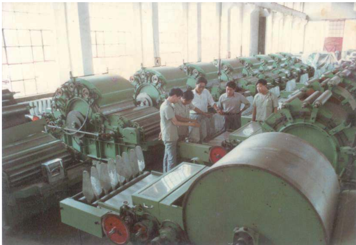
梳棉机安装车间
